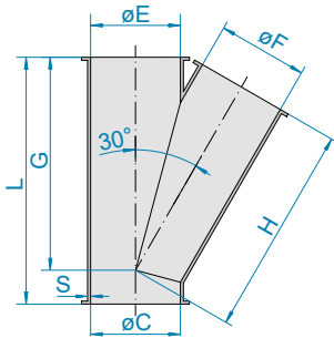
■ Lateral 30°
